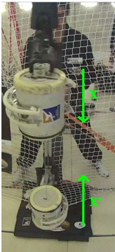
Fig. 4 – Position des axes de mesure respectif des accéléromètres par rapport au démonstrateur lors de l'expérimentation
