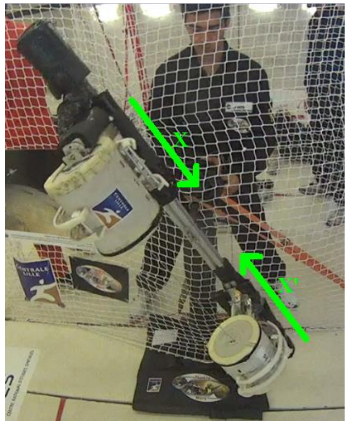
Fig. 4 – Position des axes de mesure respectif des accéléromètres par rapport au démonstrateur lors de l'expérimentation
