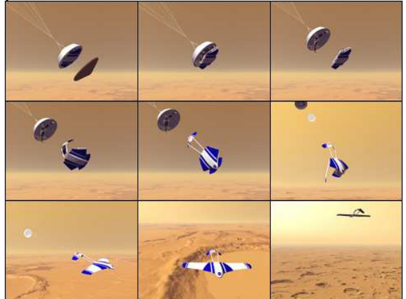
La séquence de déploiement du véhicule ARES représentée lors de sa descente dans l'atmosphère martienne. (doc. NASA)
